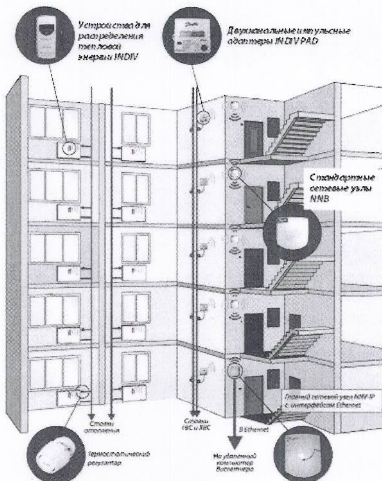
Рис.1. Структурная схема измерительной системы INDIV AMR
