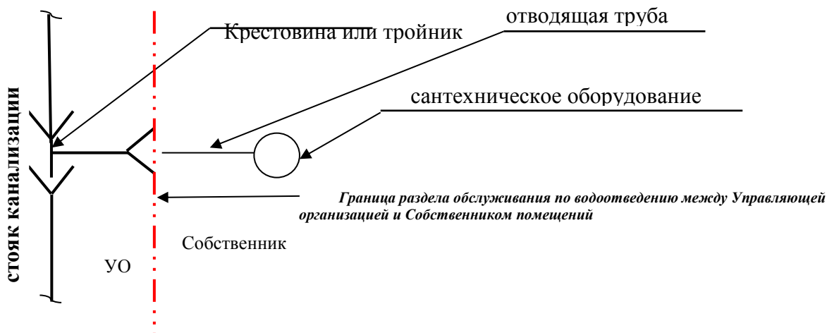
Схема № 7 Канализация
