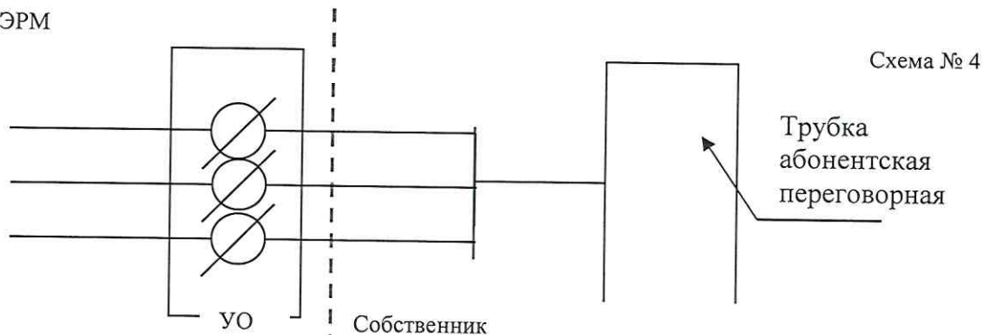
Граница раздела обслуживания по переговорному устройству домофона между Управляющей организацией и Собственником помещений
